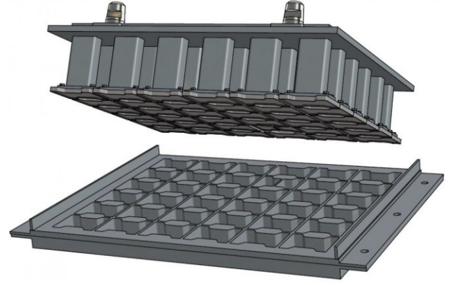
قالب ومجموعة كباسات | صورة توضيحية للمنتج
